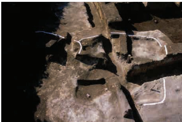
竪穴状遺構 SX61 完掘状況 (東から)
