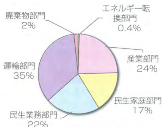
鹿児島県の二酸化炭素排出量（出典：鹿児島県）
